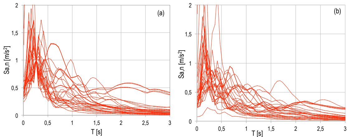
Fig. B-5 Spettri di risposta normalizzati al valore S_a(T_1)=1 : a) in direzione X; b) in direzione Y.
