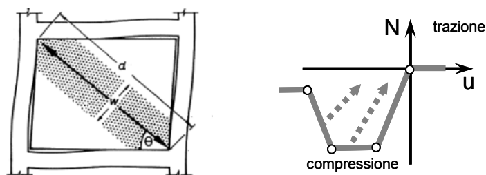
Fig. 4-8 Modelli di sezione diretti: alternative per la curva monotona (sinistra), effetto dell'interazione tra le sollecitazioni (destra).
