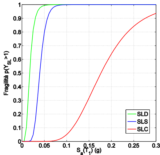
Fig. C-30 Modello B: Curve di fragilità per i tre SL.
