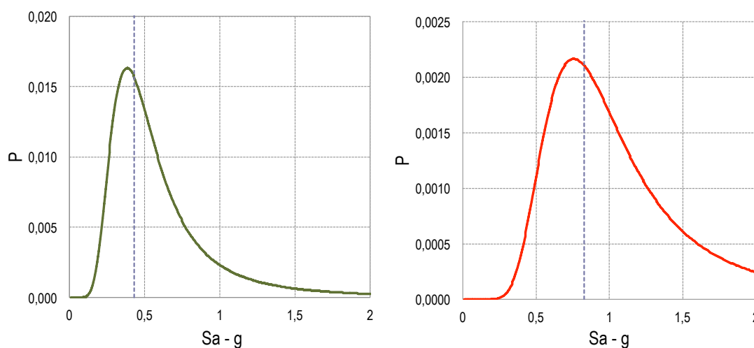
Fig. B-32 Distribuzione di probabilità condizionata per il calcolo degli stati limite SLD e SLC (è indicata la mediana della distribuzione dell'intensità sismica che porta allo SL).
